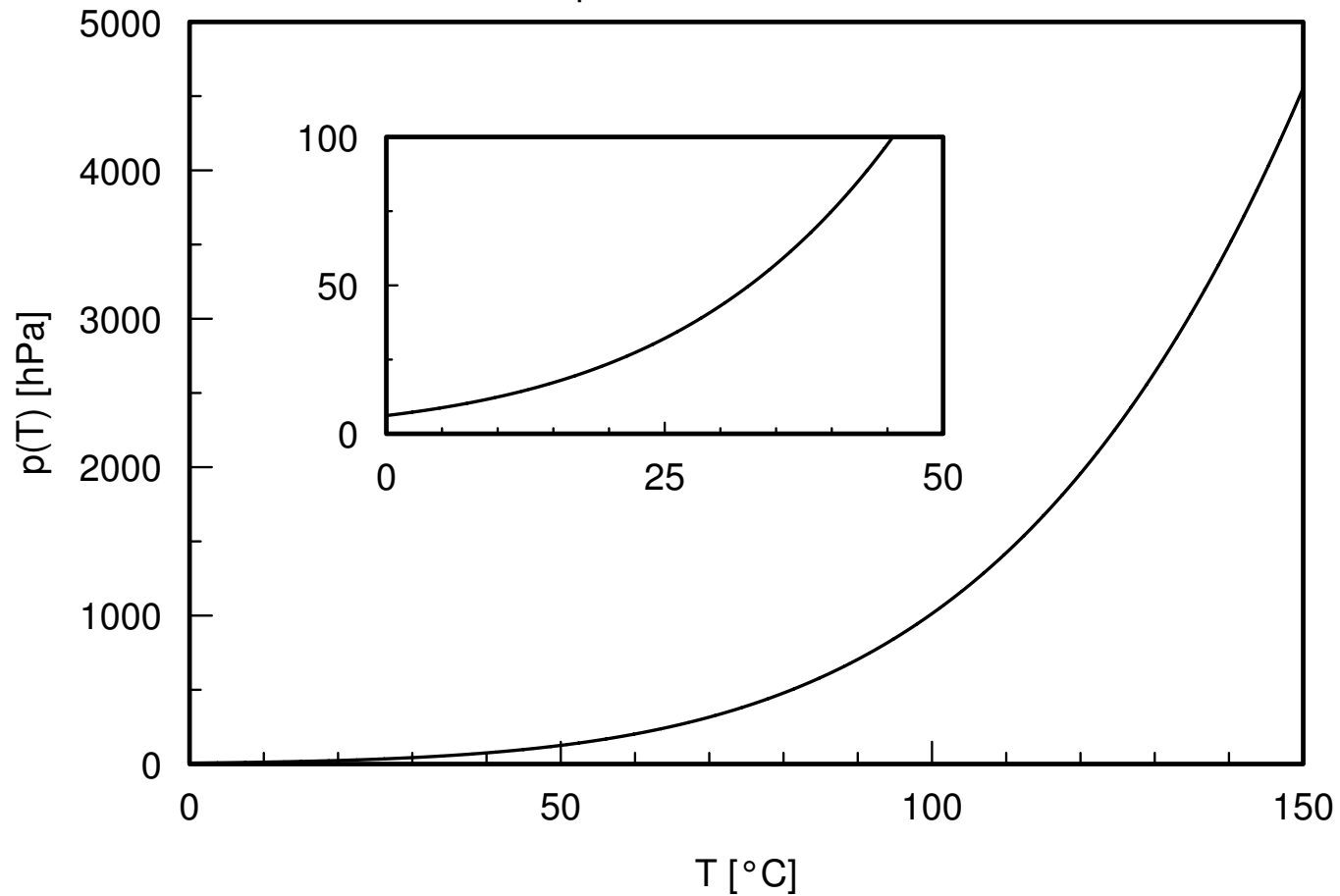
Dampfdruckkurve von Wasser
