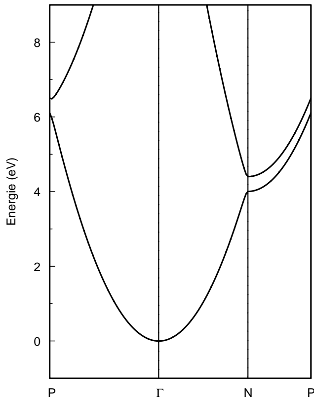
Rechnung mit 2 ebenen Wellen ( V_0=30\text{eV} )
