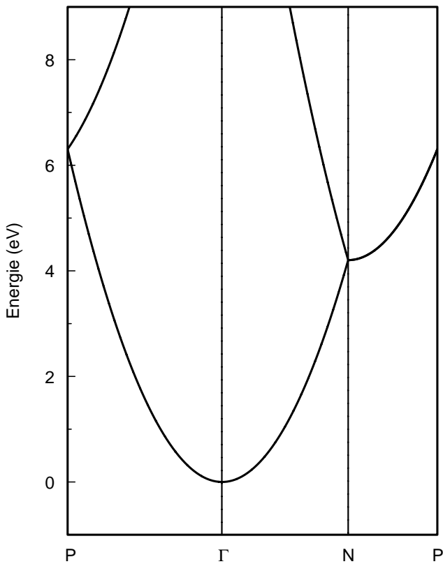
Rechnung mit 2 ebenen Wellen ( V_0=0\text{eV} )
