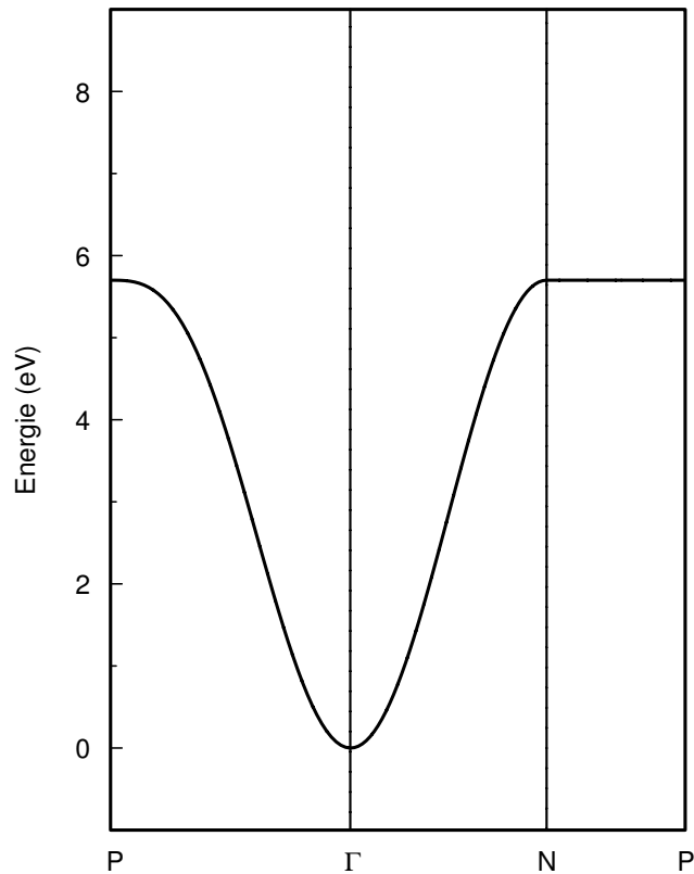
ETBM-Rechnung mit einem s-Orbital und 1.nN
